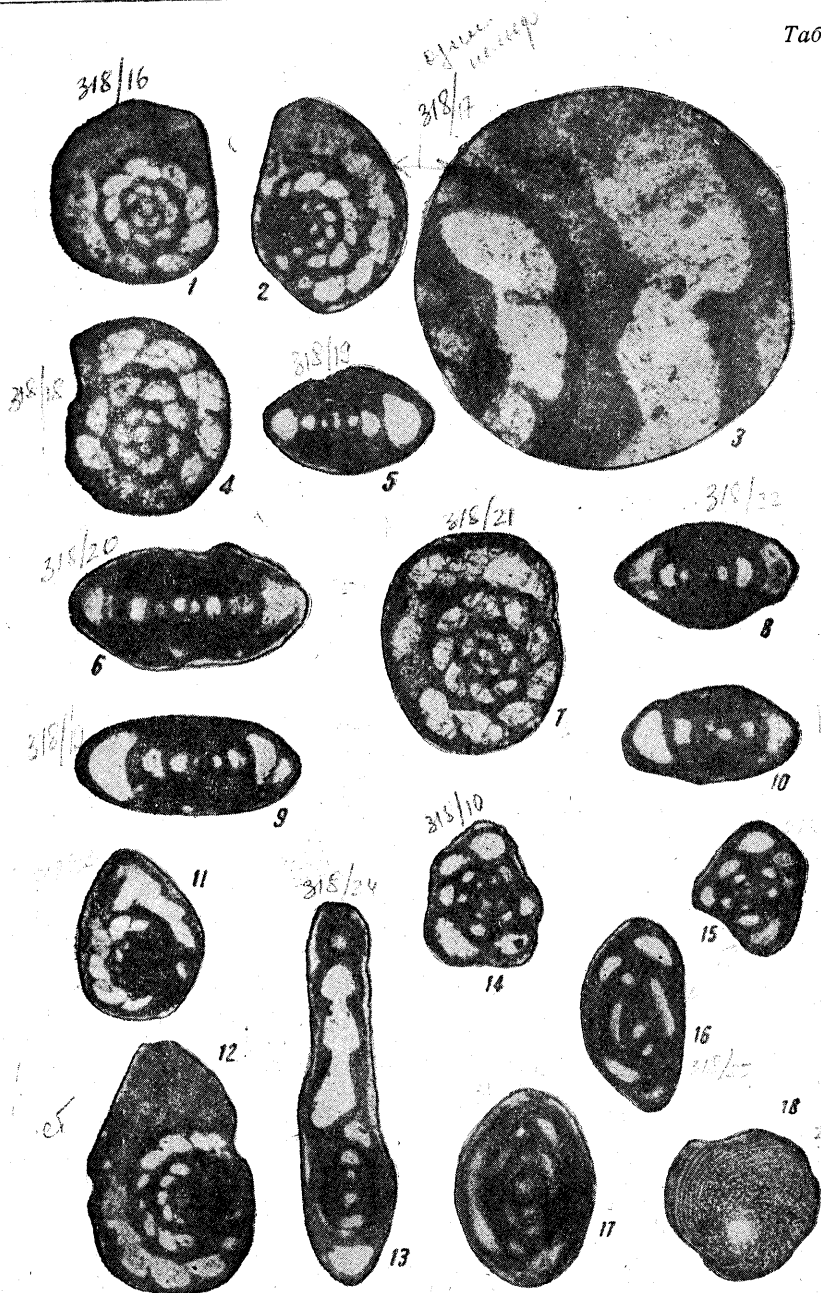
1 — 10 — Melathrokerion spiralis Gorbatchik: 1, 2, 4 — экваториальное сечение (1 = \times — 46, 2 = \times — 39, 4 = \times — 52). Юго-Западный Крым, с. Передовое. Берриас; 3 — то же, отсюда же. \times 165. Хорошо видна двухслойная стенка; 7 — экваториальное сечение, \times 64. Юго-Западный Крым, с. Глубокое. Берриас; 6, 8 — поперечное сечение (6 = \times — 43, 8 = \times — 31). Юго-Западный Крым, с. Передовое. Берриас; 5, 9, 10 — поперечное сечение (5 = \times — 51, 9 = \times — 52, 10 = \times — 45). Юго-Западный Крым, с. Глубокое. Берриас; 11, 12, 13 — Tonasia evoluta Gorbatchik: 11 — экваториальное сечение, \times 27. Юго-Западный Крым, с. Глубокое. Берриас; 12 — экваториальное сечение, \times 36. Юго-Западный Крым, с. Передовое. Берриас; 13 — поперечное сечение, \times 33. Юго-Западный Крым, с. Передовое. Берриас; 14, 15, 16, 17 — Schlumbergerina krimica Mamontova. Юго-Западный Крым, с. Передовое. Берриас; 14, 15 — поперечное сечение (14 = \times — 54, 15 = \times — 46); 16 — косое сечение, \times 37; 17 — продольное сечение, \times 53; 18 — Iberina lusitanica (Egger). Юго-Западный Крым, с. Передовое. Берриас. Экваториальное сечение \times 9.
