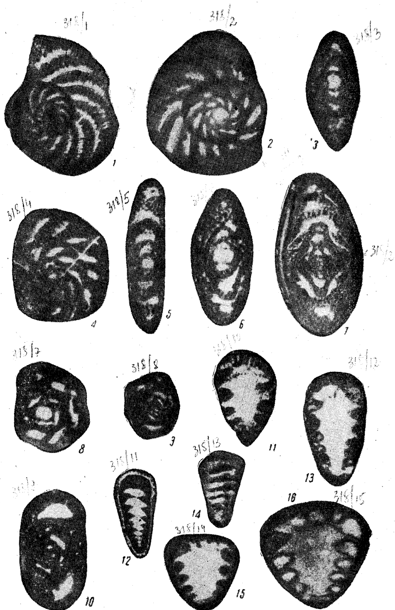
1 — 7 — Pseudocyclamina jaccardi (Schrodt). Юго-Западный Крым, с. Гончарное. Верхний оксфорд—кимеридж: 1, 2, 4 — экваториальное сечение (1 = \times —14, 2 = \times —26, 4 = \times —30); 3, 5, 7 — поперечное сечение, 8 — 10 — Pseudocyclamina sulaiyana Redmond. Юго-Западный Крым, с. Глубокое Берриас: 8, 9 — экваториальное сечение 8 = \times —25, 9 = \times —9); 10 — поперечное сечение, \times 16; 11 — 14 — Trocholina elongata (Leopold): 11 — осевое сечение, \times 16. Юго-Западный Крым, с. Передовое. Берриас; 12 — сечение, параллельное осевому, \times 13. Юго-Западный Крым, с. Глубокое. Берриас; 13 — осевое сечение, \times 23. Юго-Западный Крым, с. Глубокое. Берриас; 14 — внутренний вид половины раковины. Хорошо видно внутреннее спиральное ребро, \times 16. Юго-Западный Крым, с. Глубокое. Берриас; 15 — 16 — Trocholina alpina (Leopold). Юго-Западный Крым, с. Передовое. Берриас; 15 — осевое сечение, \times 24; 16 — осевое сечение, \times 27.
